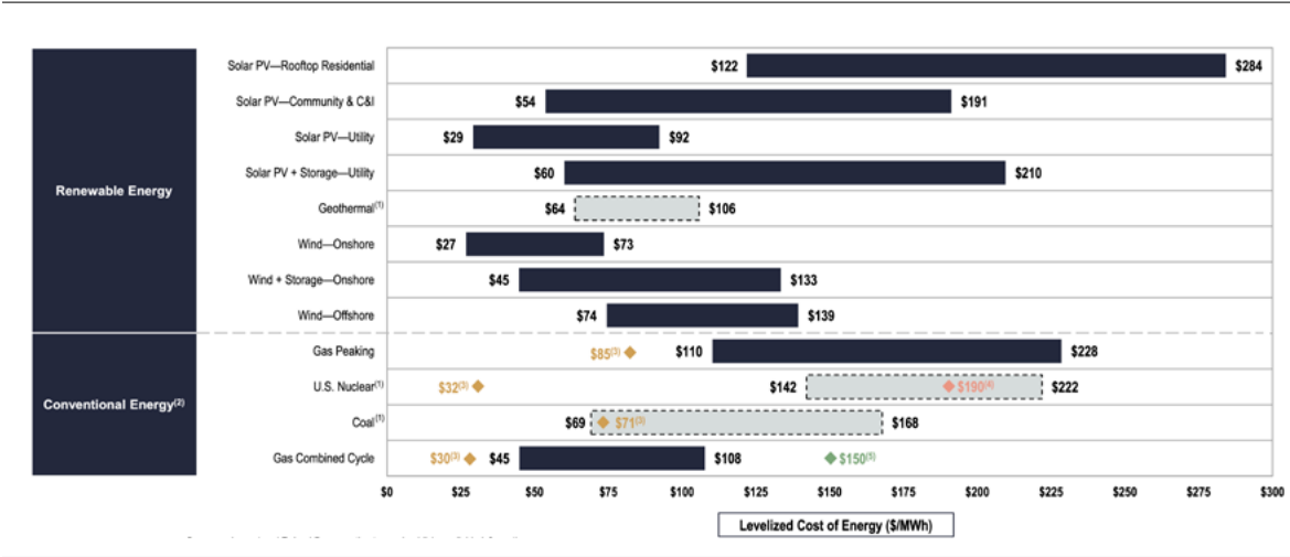
Figure 5 – Coût actualisé de l'énergie pour diverses productions. En orange : les coûts de production une fois les coûts d'infrastructure amortis.
